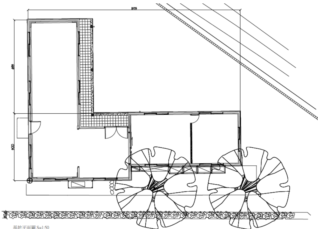
圖 1 基地平面圖
